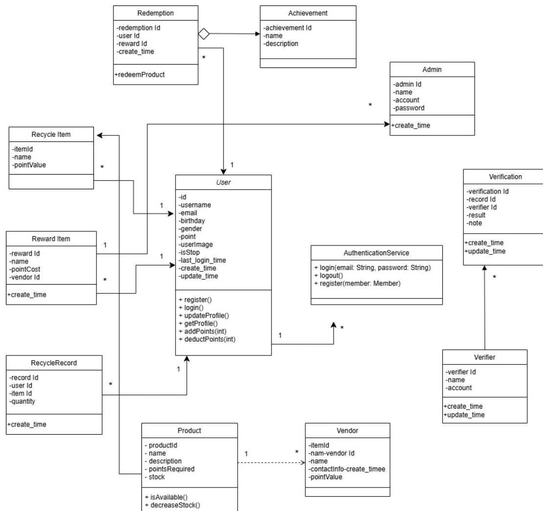
圖 6-2-1 設計類別圖
