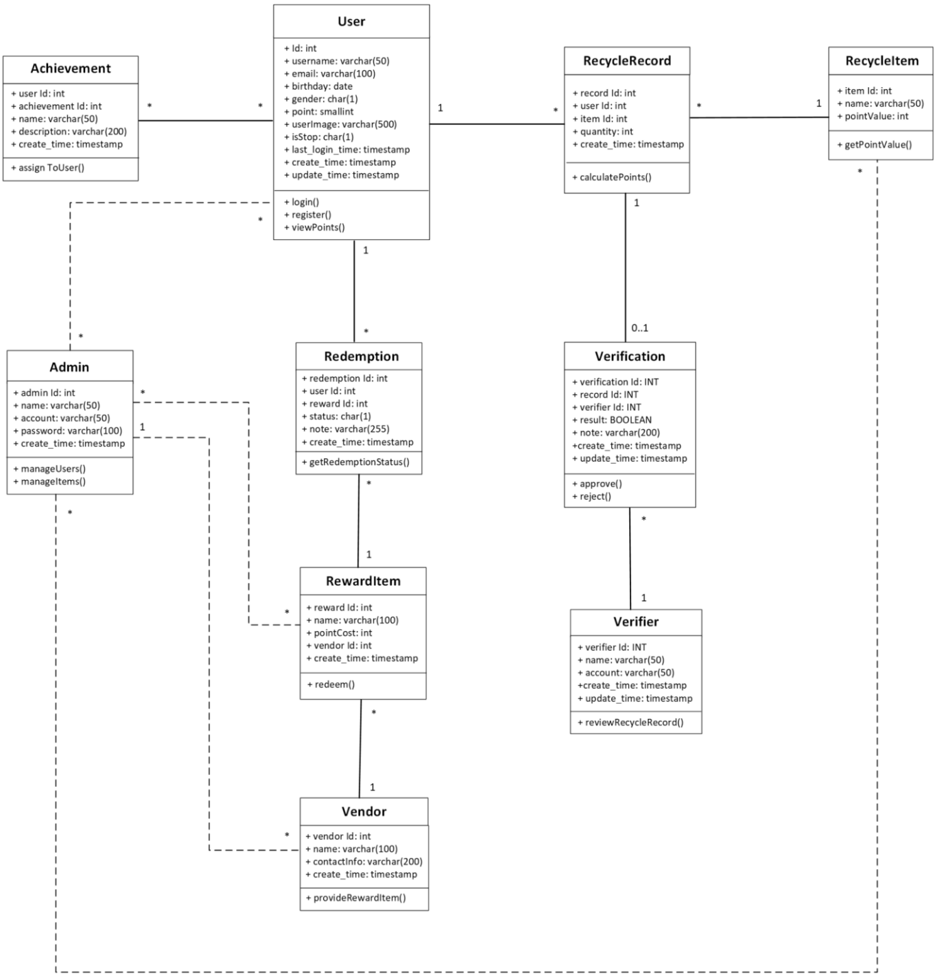
圖 5-4-1 分析類別圖
