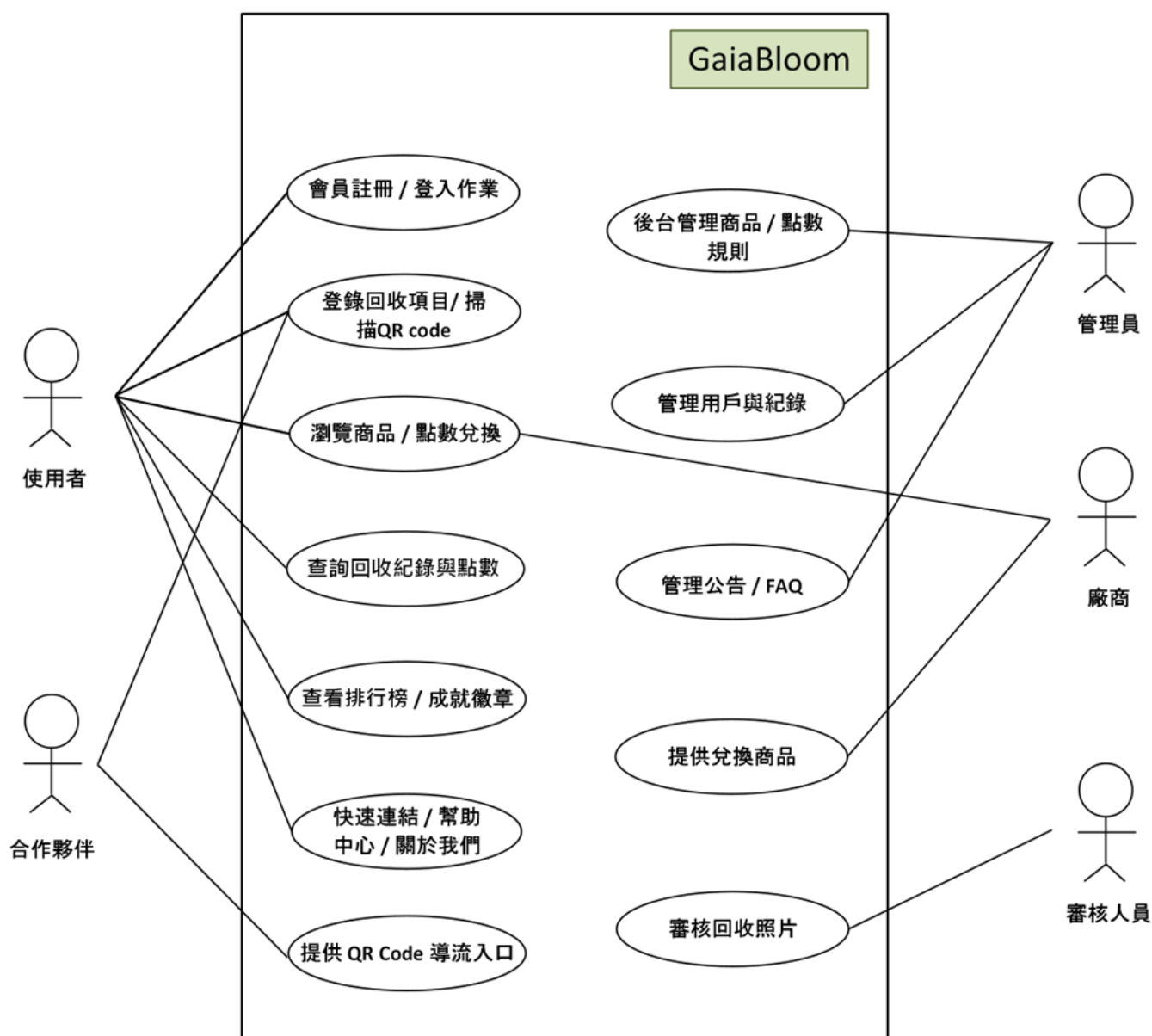
圖 5-2-1使用個案圖
