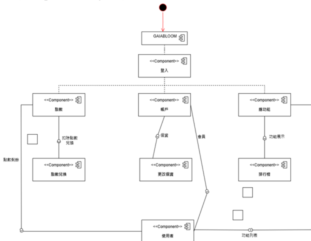
圖 7-3-1 元件圖
